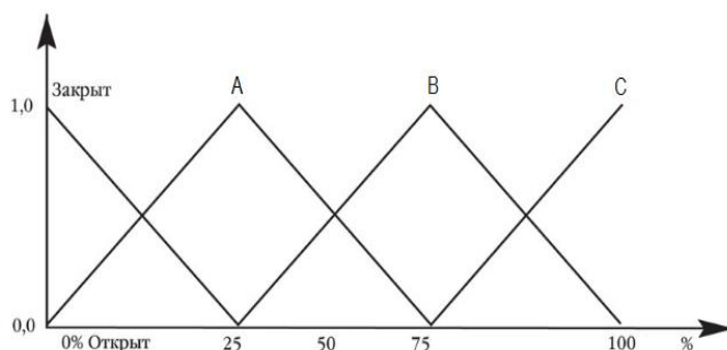
Рис. 2. Описание работы нечеткого клапана
